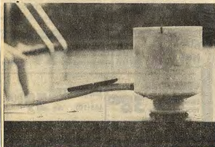
Vågenergipumpen är ca 25 cm hög och väger ett halvt kilo. Båtägaren gör bara ett hål i botten på båten, sätter fast pumpen och lägger ut slangen i kölsvinet. Vågenergin räcker för att redan i en förtöjd båt pumpa ut nära fyra liter i minuten
