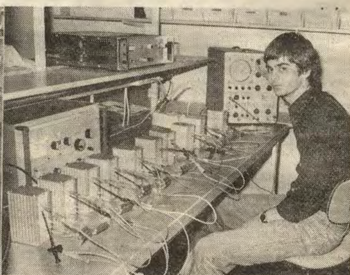
Mats Johansson tittar till ett långtidsprov av tio prototyper, som tagits fram av SJ och nu skall testas i kommunikationsradioanläggningar på tågen
