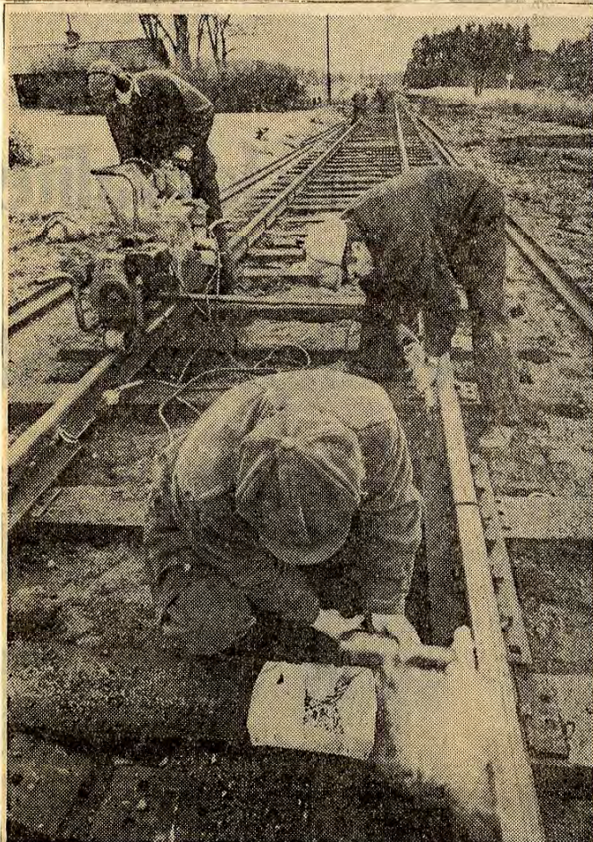
25 man är sysselsatta med att byta räls och slipers
